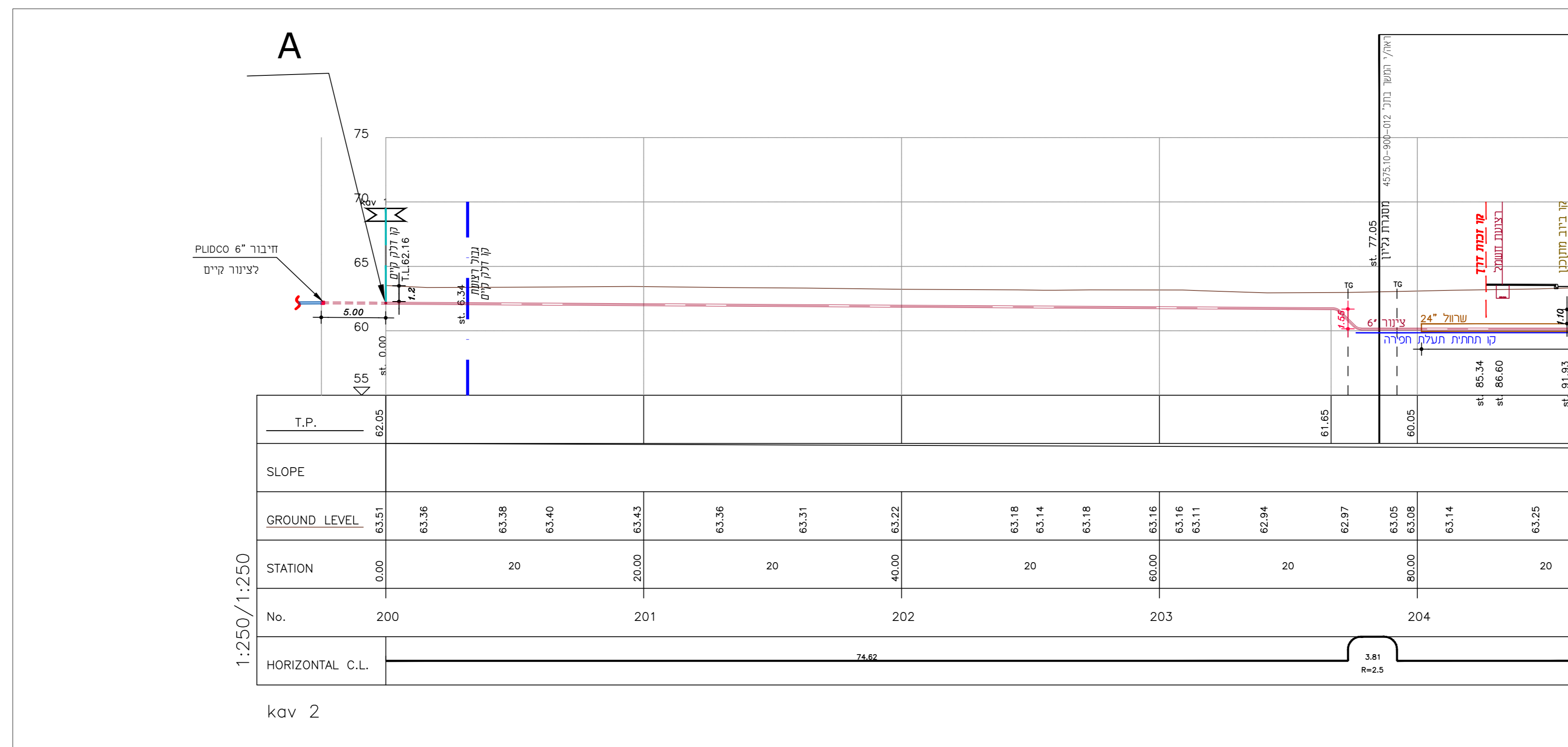
חתך לאורך מסי 1 1:250/1:250
